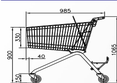
ATC 150
