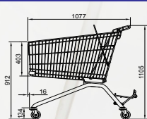
ATC 210 L
