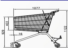
ATC 210
